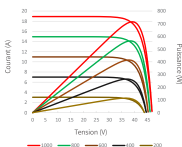
Courbes courant-tension et puissance-tension (700W)
